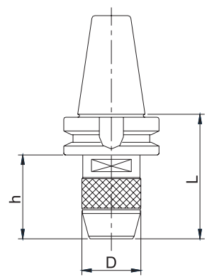
MANDRENLİ BAŞLIK
